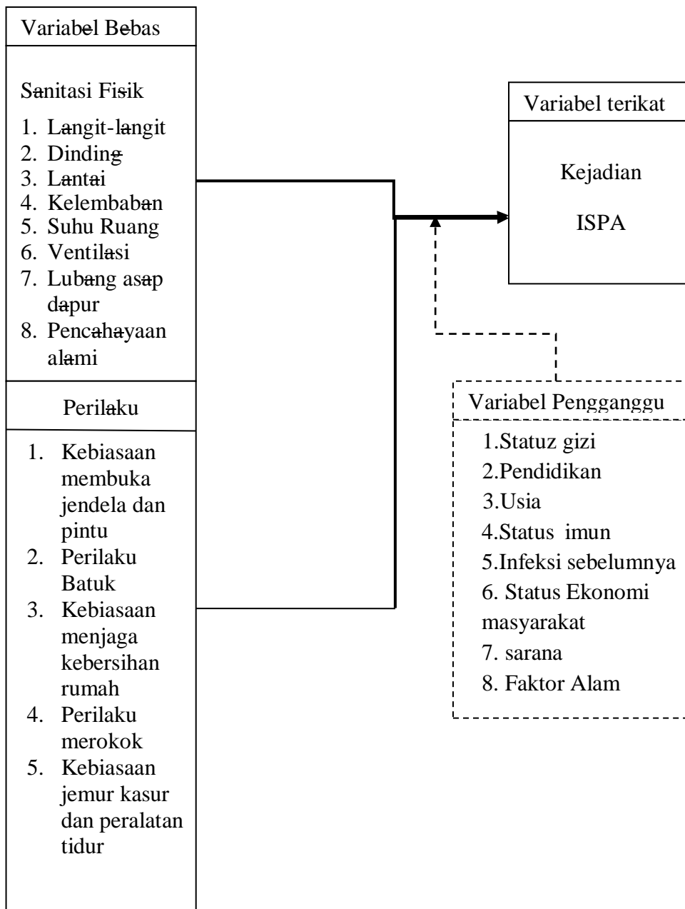
Gambar III.2 Kerangka Konsep
