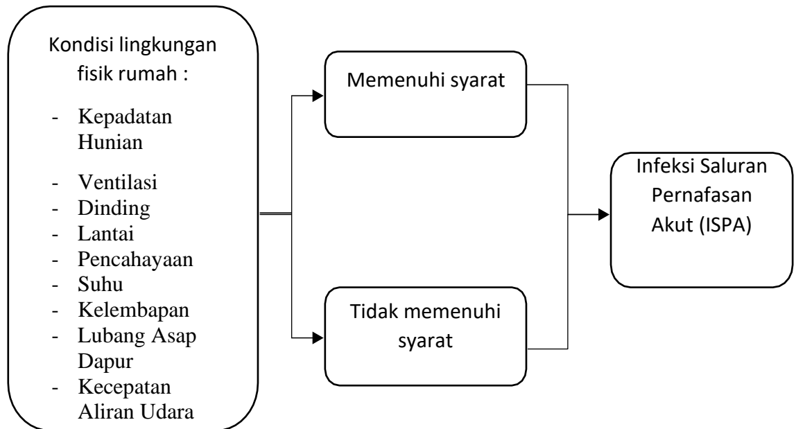
Gambar II.2 Kerangka konsep
